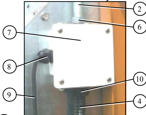
Plenum high limit thermo.
