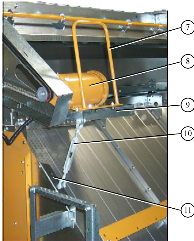
Top Auger motor and motor mount.
