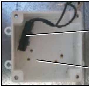
Plenum high limit conduit (plenum pipe).
