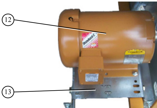
Bottom Auger motor and motor mount.
