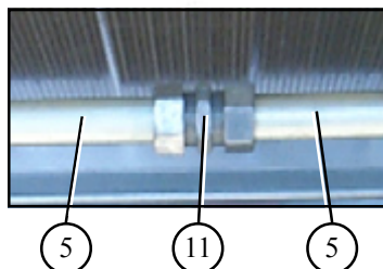
Coupler for 1/2" EMT conduit.
