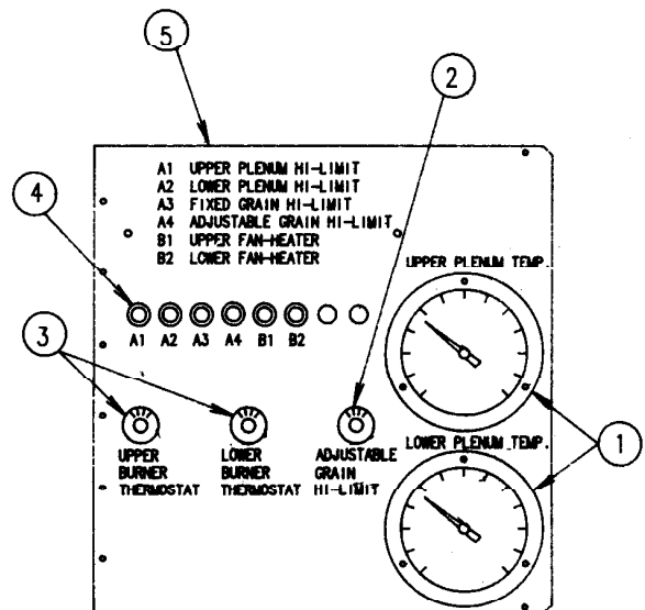
1500LS MODULE
