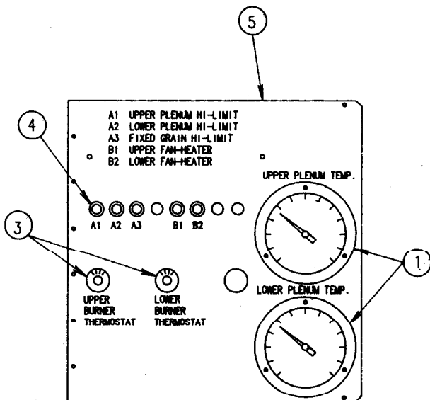
750LS MODULE
