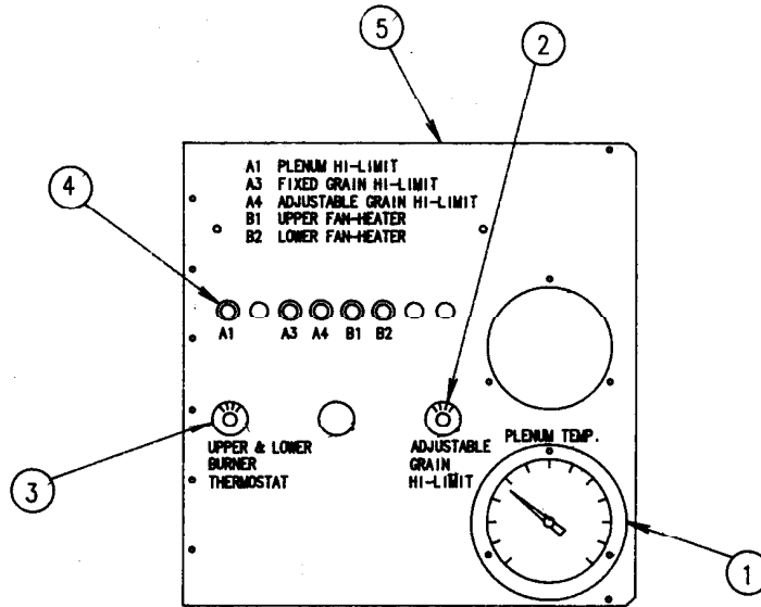
2300LS MODULE
