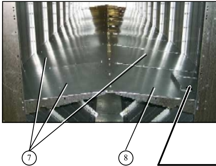
Plenum divider.
