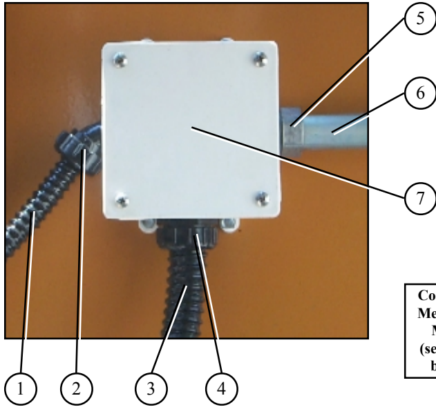
Meter roll motor conduit connection.
