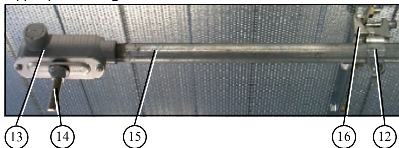
Upper plenum high limit thermostat conduit.
