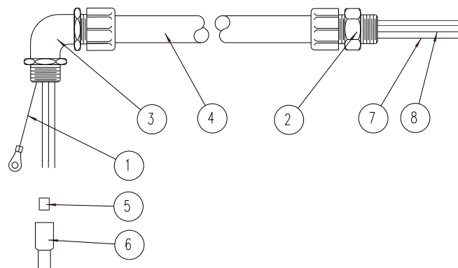
C-8264 CONDUIT ASY-3/4"X3"STR/ELB 1PH
